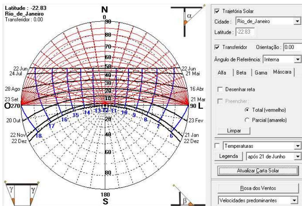
Figura 4.12 - Trajetória solar
