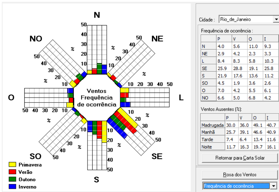
Figura 4.10 - Direção predominantes dos ventos segundo estação do ano
